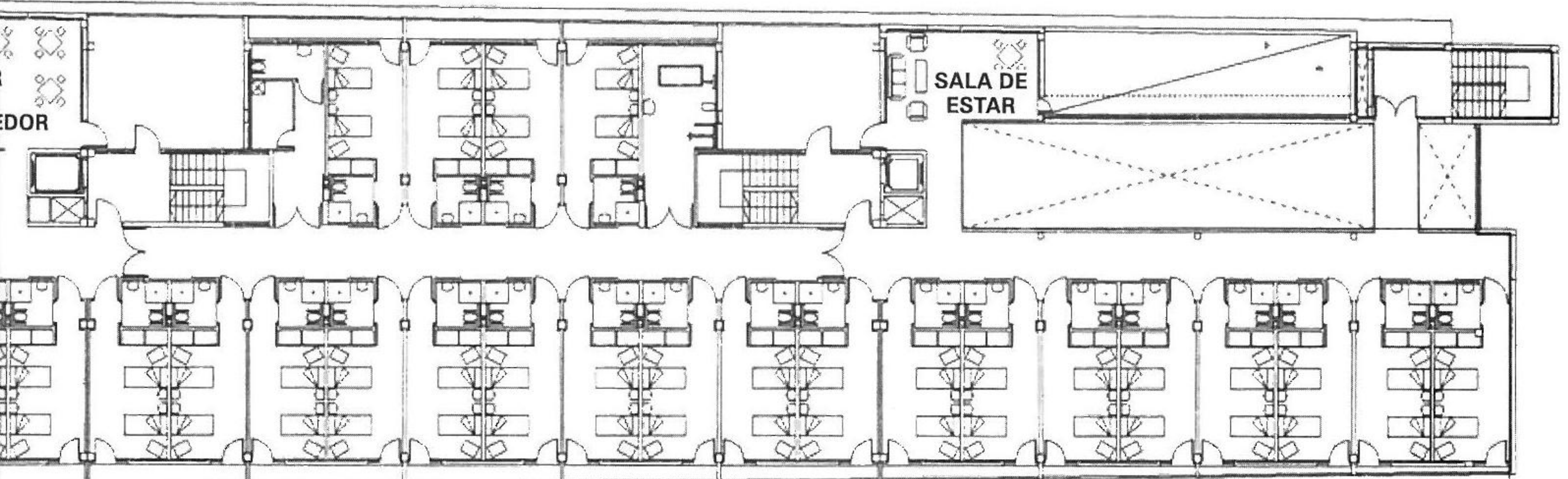
PLANTA PRIMERA Y SEGUNDA - HABITACIONES
